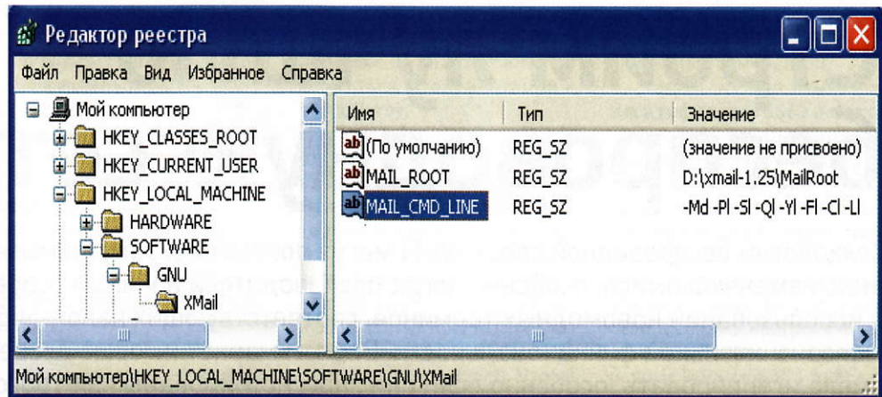
Рис. 2. Запустите редактор реестра. Создайте ветку HKEY_LOCAL_MACHINE\SOFTWARE\GNU\XMail со строковыми параметрами MAIL_ROOT = "D:\xmail-1.25\MailRoot" и MAIL_CMD_LINE = "-Md -PI -SI -QI -YI -FI -CI -LI"
